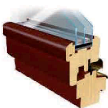
Profiel met driedubbel beglazing en speciaal vorm van de laat.
